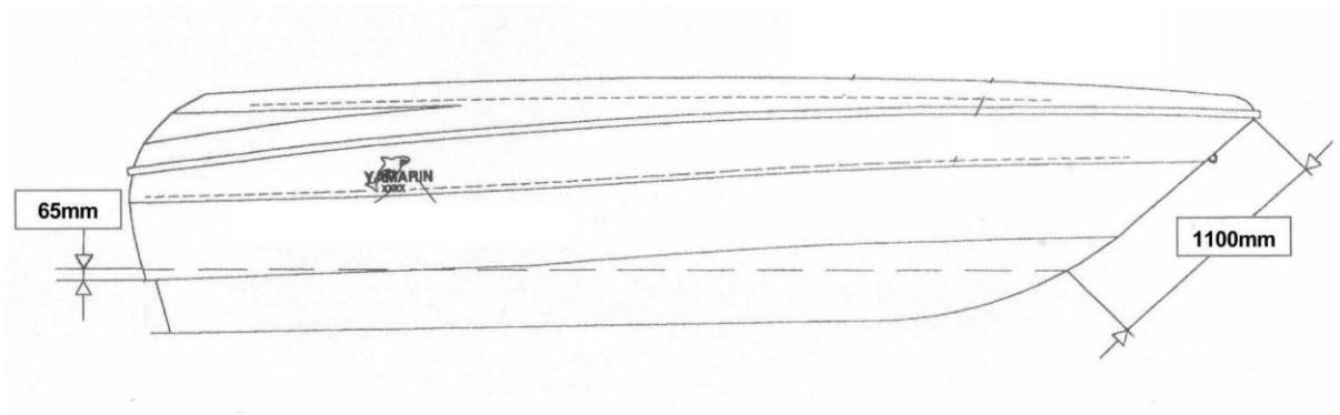
Ватерлиния судна Yamarin 59 Day Cruiser
