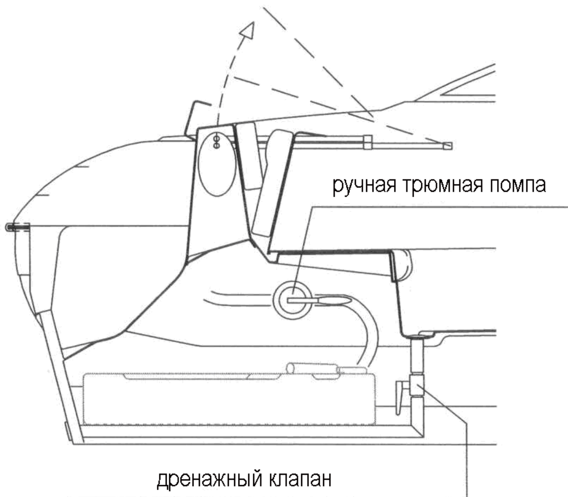
Расположение кингстонов и сливных клапанов на судне Yamaha 59 Day Cruiser
